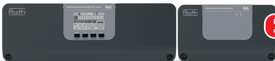
Roth Touchline® SL kontrolenhed, 12 kanaler 8+4 VVS-nr. 466397.062
